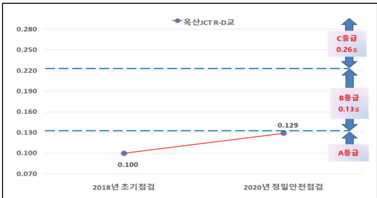
[그림 3.4.1] 옥산JCT R-D교 상태평가 결과 비교 그래프
